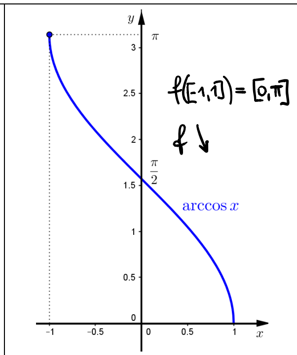
Funzione arcocoseno f(x) = \arccos x , x \in [-1, 1]
