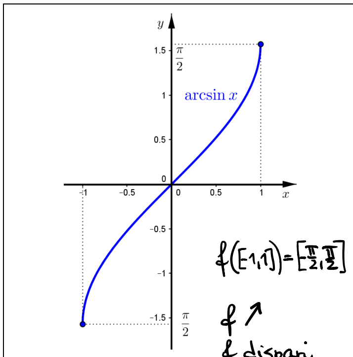
Funzione arcseno f(x) = \arcsin x , x \in [-1, 1]
