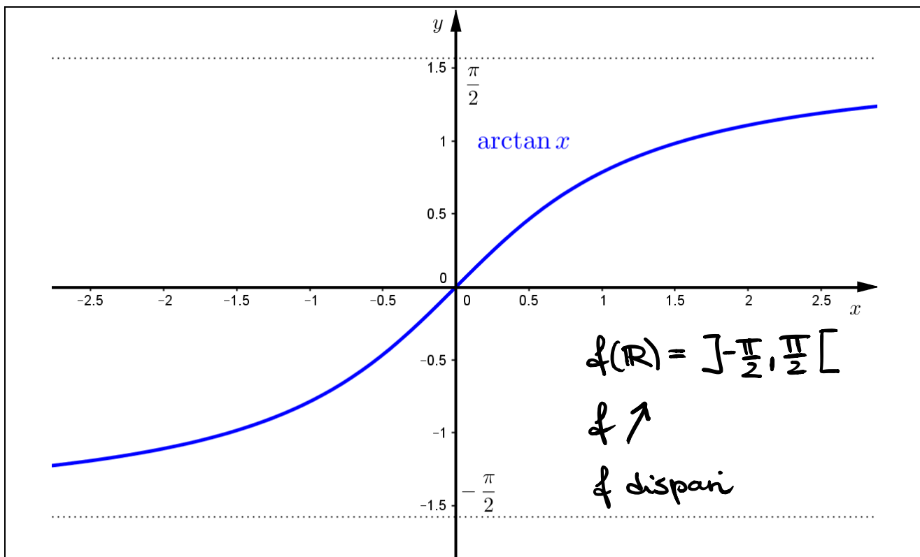
Funzione arcotangente f(x) = \arctan x , x \in \mathbb{R}
