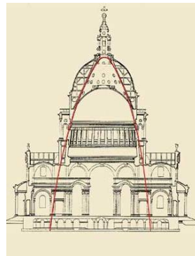
Cupola di Saint Paul (Robert Hooke), Londra
